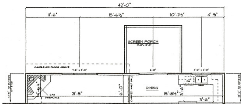
OPTIONAL SCREEN PORCH
